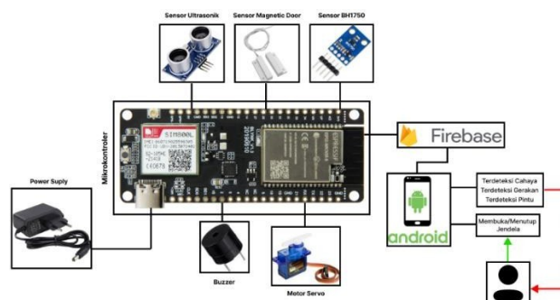
Gambar 2. Gambaran Umum Sistem
